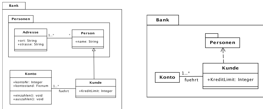
Abbildung 8: Semantische Fokus-und-Kontext-Darstellung eines Diagramms nach Koeth [17].
